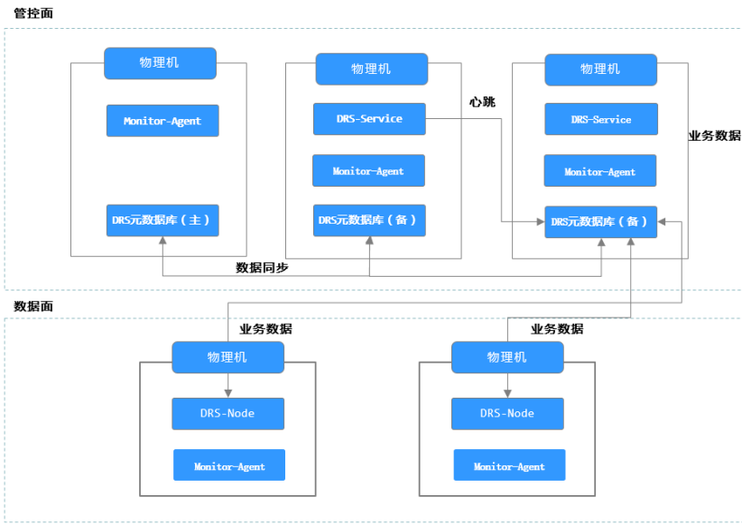
图 1-3 DRS 高可用部署架构
